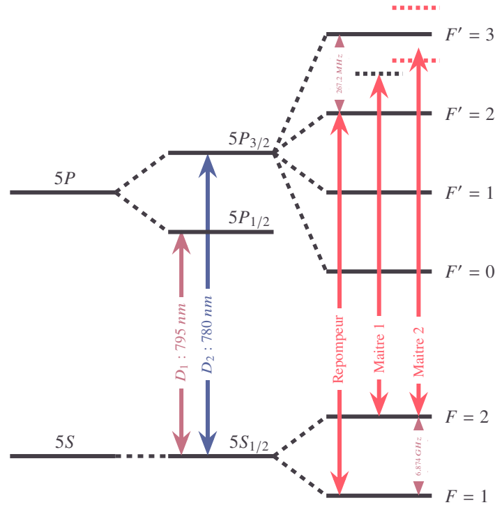
FIGURE 5.1 – Structure hyperfine (transitions D1 et D2) de l'atome de Rubidium ^{87}\text{Rb} . Les longueurs d'onde de différents lasers utilisés dans l'expérience sont représentées en rouge vif
