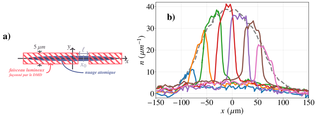
FIGURE 5.5 – (a) Schéma illustrant la sélection d'une région du nuage atomique, ici représentée par une ellipse bleue illuminée par un faisceau modulé à l'aide du DMD . (b) Exemple de sélections sur un gaz initialement à l'équilibre : superposition du profil de densité initial du nuage (courbe grise) et des profils mesurés après \tau = 1\text{ ms} pour différentes régions de sélection de taille \ell = 37\mu\text{m} centrées en différentes positions x_0 (courbes colorées).
