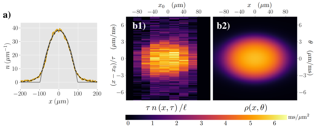
FIGURE 5.6 – a) Profil de densité d'un nuage atomique initialement à l'équilibre dans un piège harmonique avec \omega_{\perp} = 2\pi \times 2.6\text{ kHz} et \omega_{\parallel} = 2\pi \times 5\text{ Hz} (jaune). La courbe grise représente le profil parabolique attendu à l'état fondamental dans le régime qBEC , décrit par l'équation d'état n(x) = [\mu - V_{\parallel}(x)]/g . La courbe noire en pointillés correspond à un ajustement des données expérimentales en supposant que le système soit bien décrit par un ensemble thermique ( TBA (Sec. 2.2.2)). Cet ajustement permet d'extraire une température T = 90\text{ nK} et un potentiel chimique \mu/k_B = 49\text{ nK} . (b1) Profils de densités pour différents centres de sélection x_0 représentés sur la Fig.5.5(b). Les sélections sont de taille \ell = 37\mu\text{m} et les profils obtenus après un temps d'expansion \tau = 40\text{ ms} . Pour comparer les résultats à une distribution de rapidités, les profils de densités sont multipliés par le rapport \tau/\ell et sont tracés en fonction de (x - x_0)/\tau . (b2) Prédiction théorique de la distribution de rapidités spatialement résolue \rho(x, \theta) à l'équilibre thermique dans un potentiel harmonique longitudinal avec \omega_{\parallel} = 2\pi \times 5\text{ Hz} . La température T et le potentiel chimique \mu utilisés sont ceux obtenus à partir du profil in situ (a).
